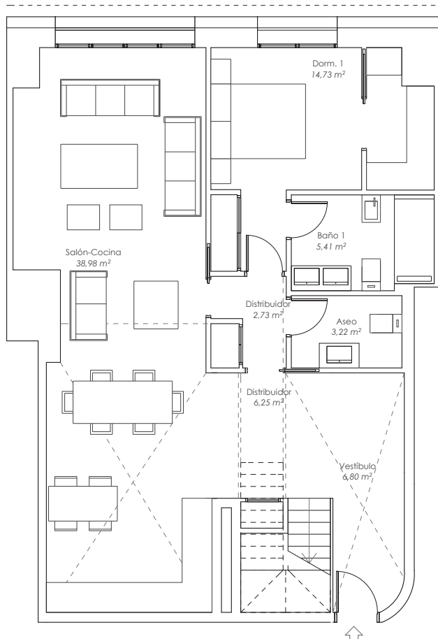
PLANTA 2ª
