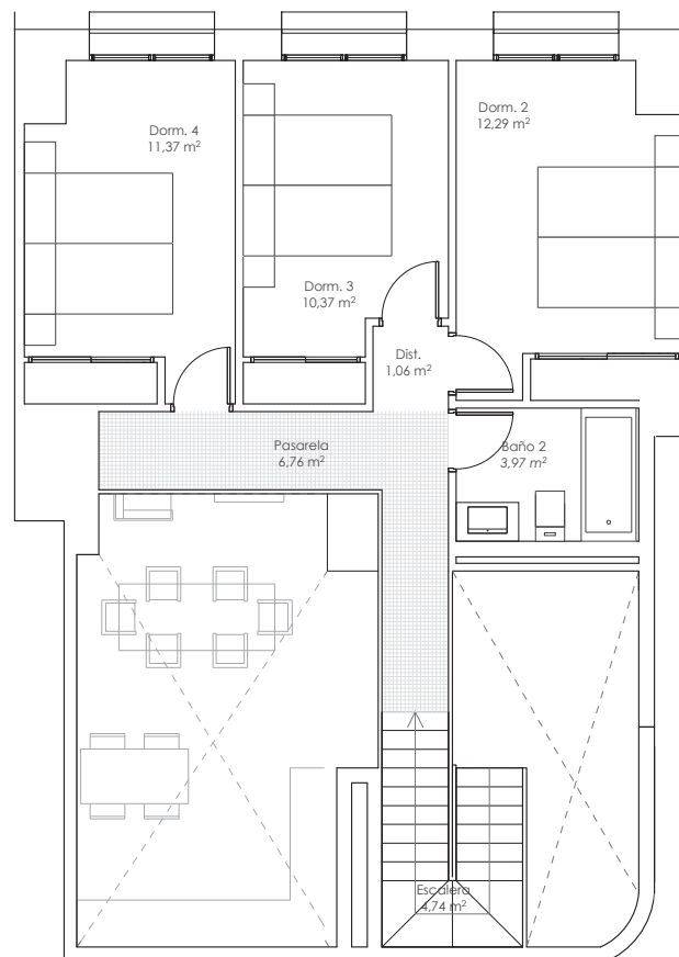
PLANTA 3ª
