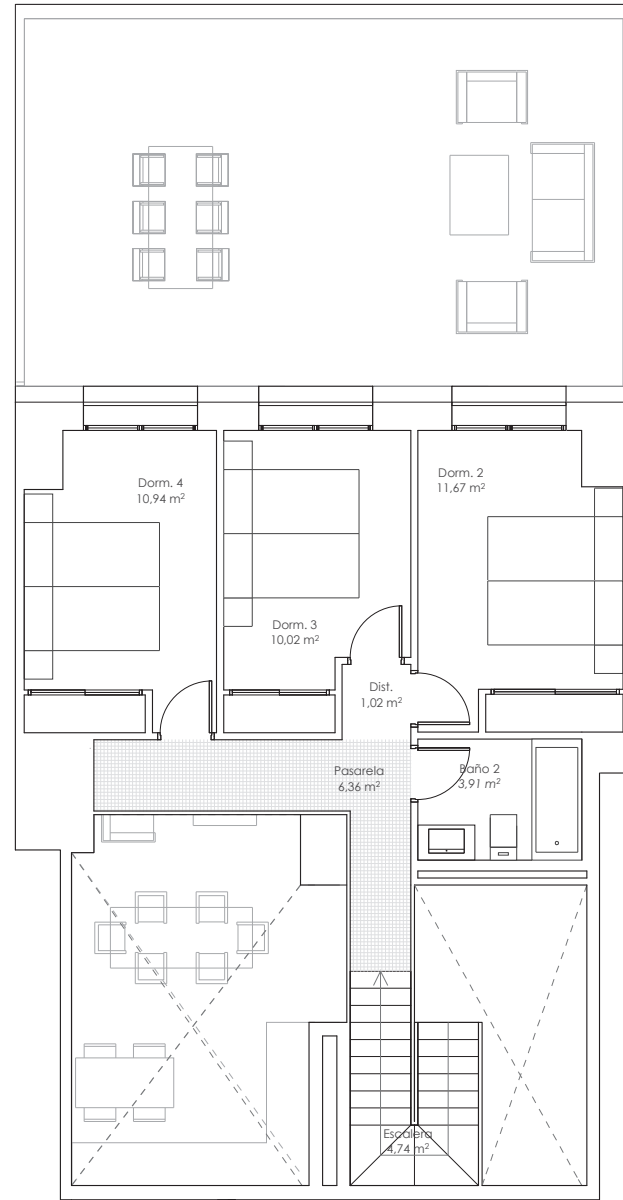
PLANTA 1ª
